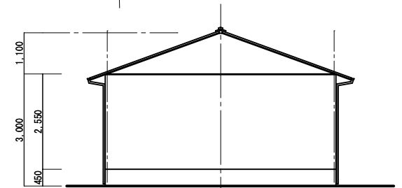
東側立面図 1:100
