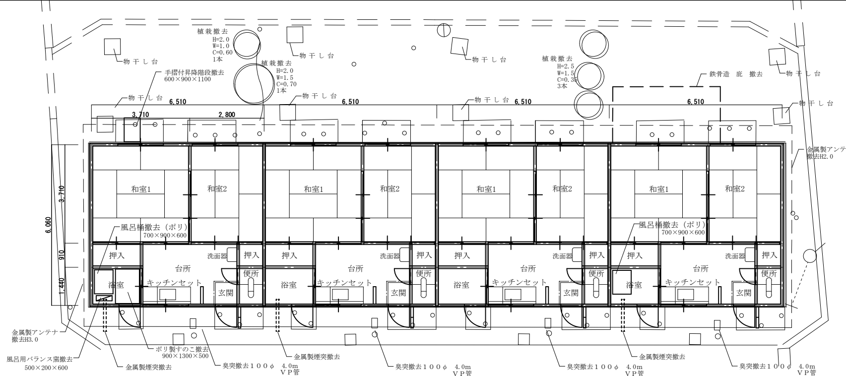
平面図 1 : 100
