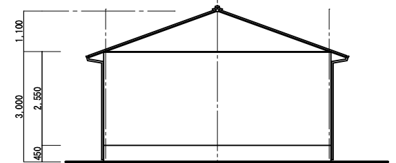
西側立面図 1:100
