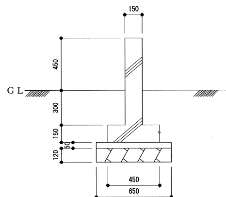
一般布基礎
