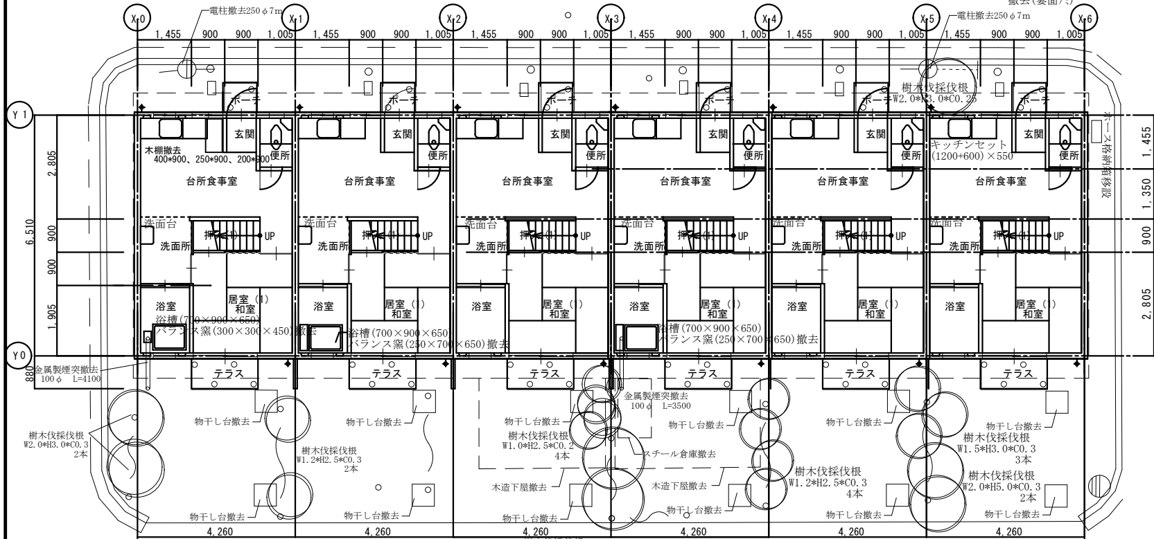
1階平面図 1:100
