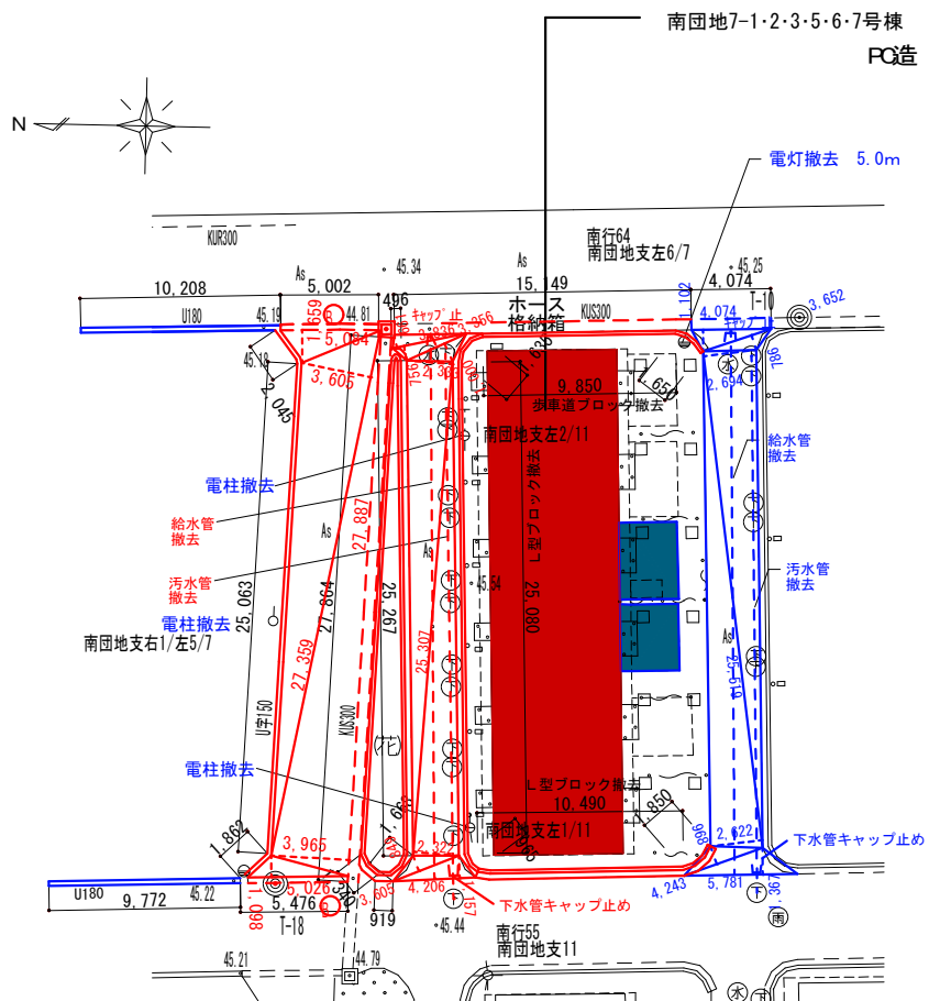
外構図 1: 300
