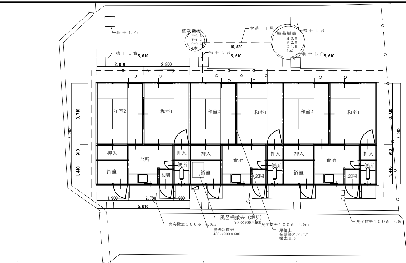
平面図 1:100
