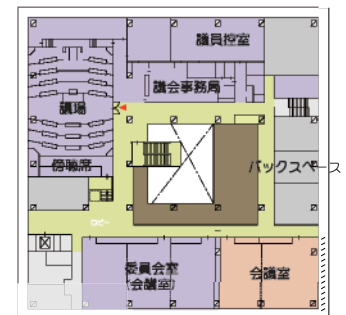
3階平面図
