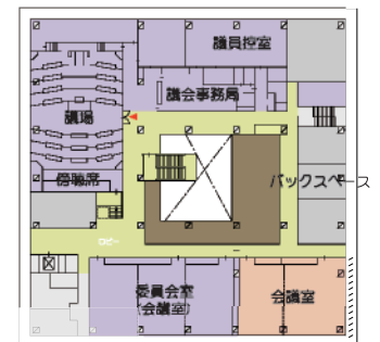
3階平面図
